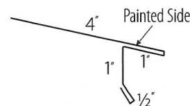
DRIP EDGE
